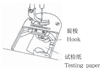
第1图 加油状态的调查方法 Fig.1:How to check state of lubrication
